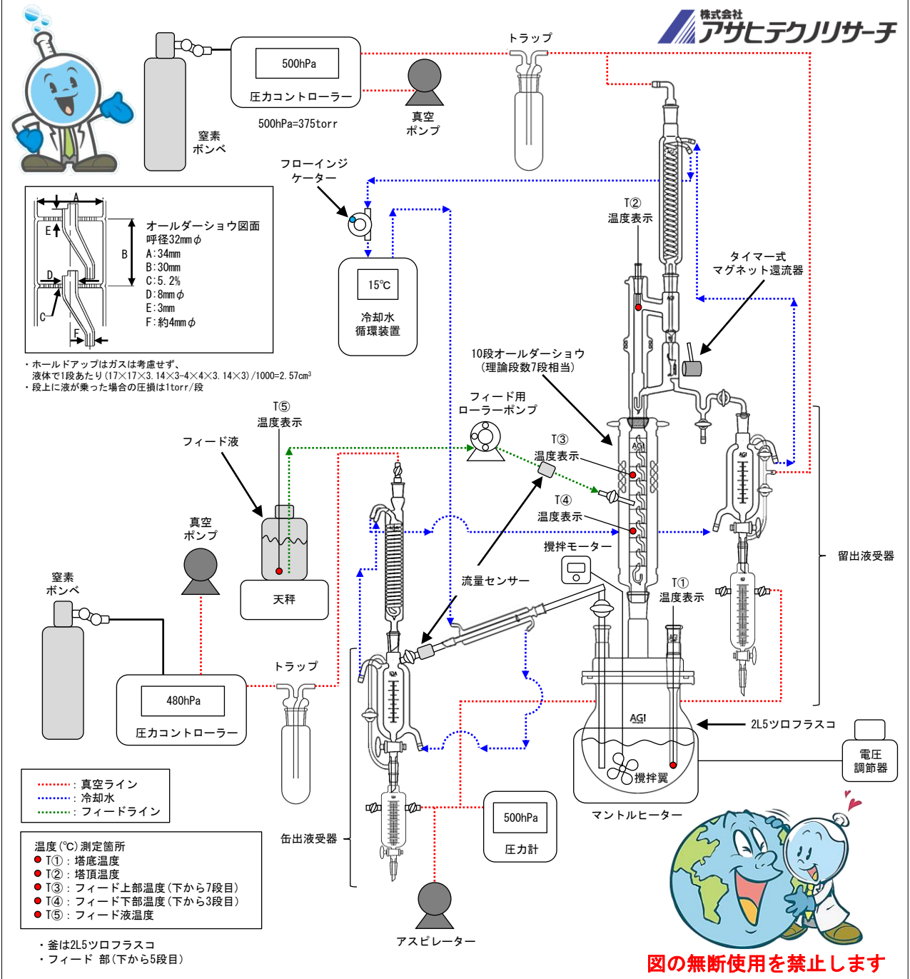
ガラス製蒸留装置イメージ図-4 (オールダーショウ10段×1本 連続蒸留/減圧系)
