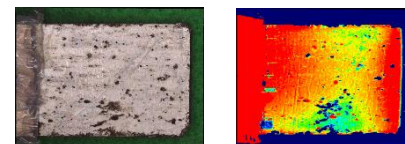
腐食状況の3D解析
