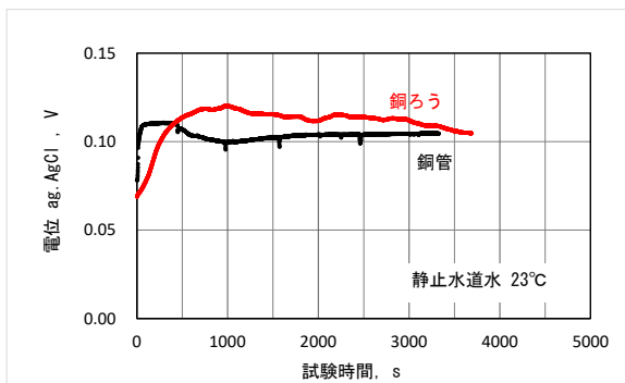
銅-銅ろうのガルバニック腐食検証試験
