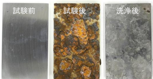
乾湿繰り返し試験
