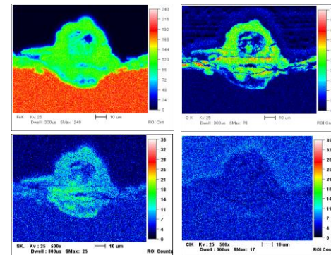
面分析による腐食成分の分布
