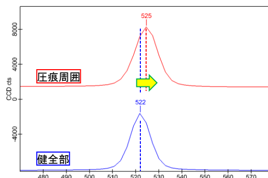
圧縮応力によりピークが高波数側にシフト
