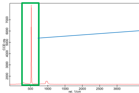
シリコンウエハーのRamanスペクトル
