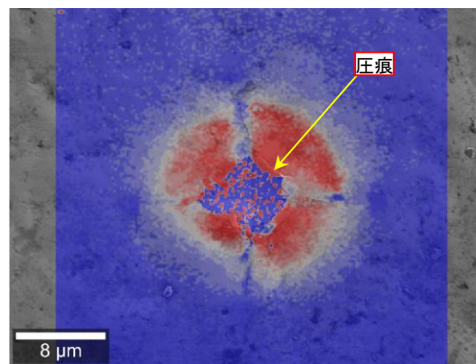
SEM画像とRamanマッピングの合成
