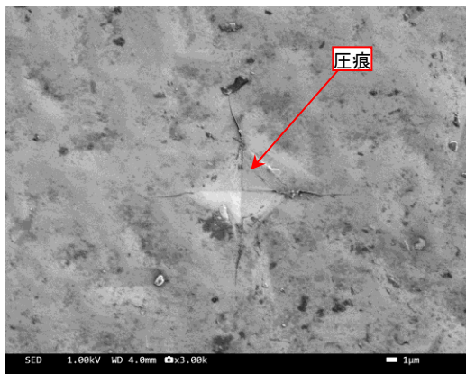
シリコンウエハー上のビッカース硬さ圧痕
